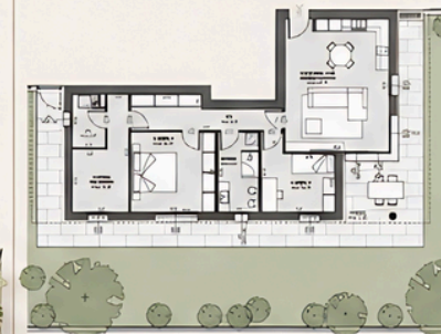
Planimetria di progetto
