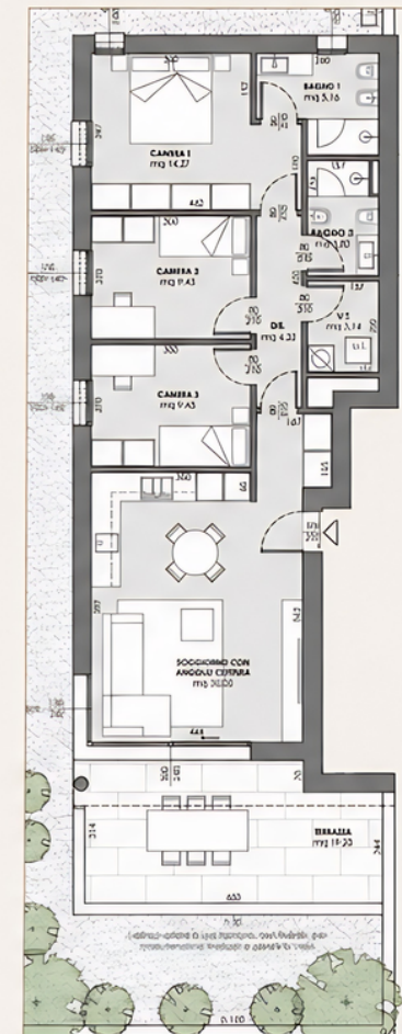
Planimetria di progetto
